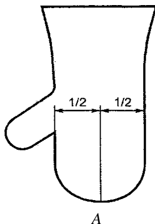
Рисунок 1 – Подвешивание перчатки для испытания
